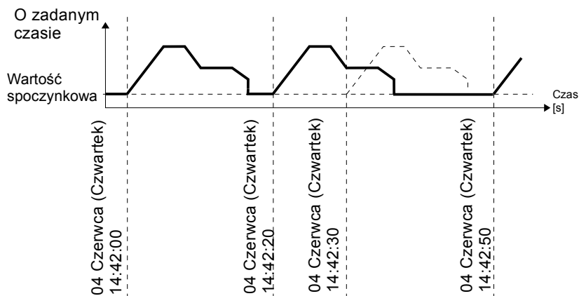
Rys.7.119. Przebieg sygnału wyjściowego dla trybu o zadanym czasie i parametrów czasowych zgodnych z Rys.7.118
