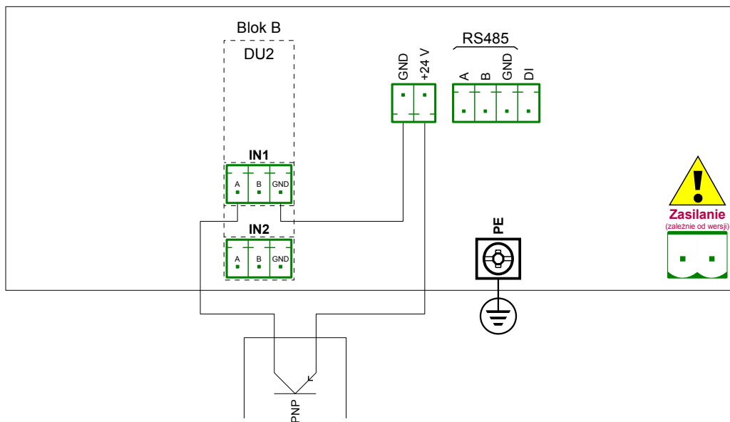
Rys. 8.10. Schemat podłączenia czujnika z wyjściem typu PNP do konfiguracji sprzętowej DU2
