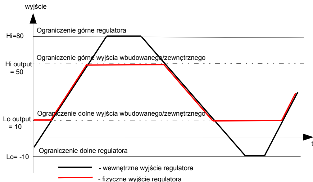
Rys. 7.132. Ograniczenia wyjścia pętli sterującej
