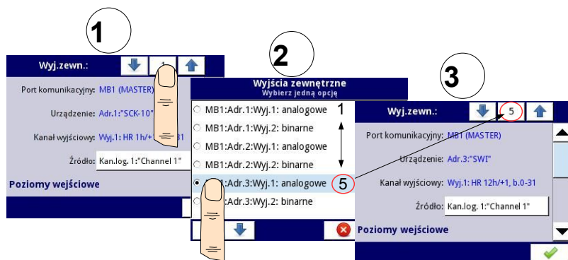
Rys. 7.108. Widok przykładowego Wyjścia zewnętrznego w konfiguracji jako wyjście liniowe (analogowe)
