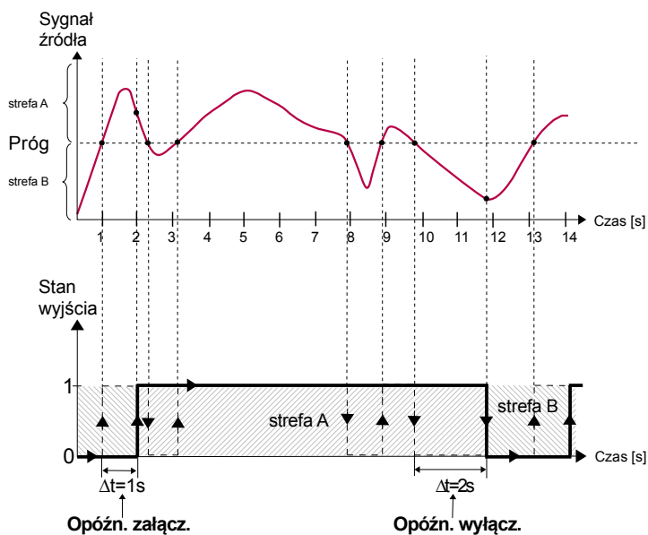
Rys. 7.97. Zasada pracy przełączników wirtualnych dla przykładowych ustawień czasowych: Opóźn.załącz. = 1 sec., Opóźn.wyłącz. = 2 sec.
