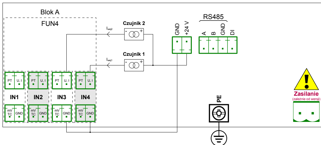
Rys. 8.4. Podłączenia przetworników prądowych 2-przewodowych
