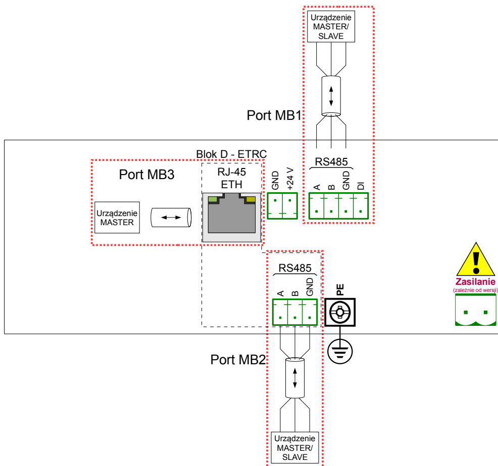
Rys. 7.163. Szeregowe porty komunikacyjne dostępne w urządzeniu
