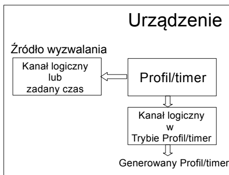
Rys. 7.112. Schemat blokowy konfiguracji urządzenia przy generowaniu Profili/timerów
