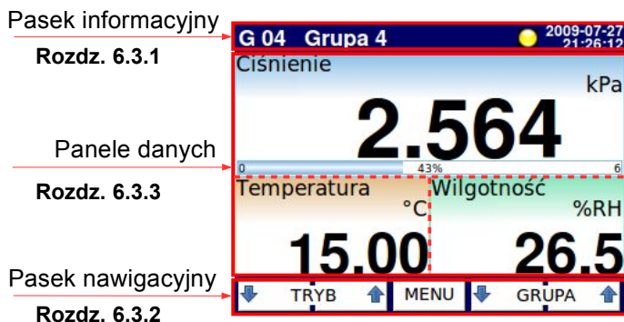
Rys. 6.4. Widok wyświetlacza MultiCon CMC-N16 po dotknięciu ekranu w czasie normalnej pracy urządzenia
