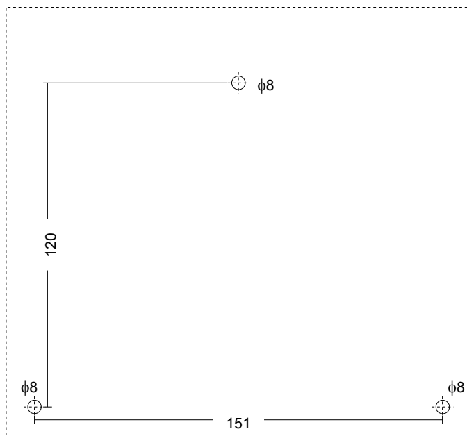
Rys. 4.2. Rozmieszczenie otworów montażowych w ścianie
