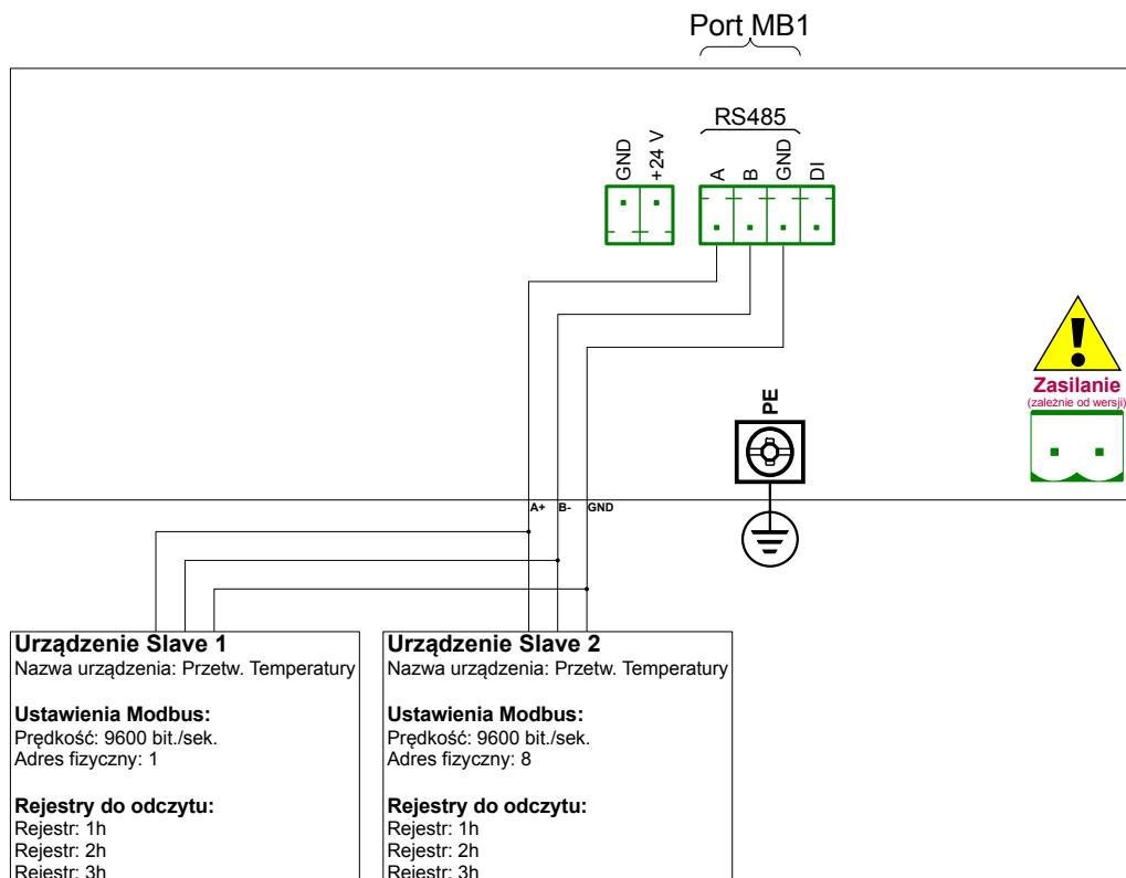
Rys. 7.167. Schemat połączeniowy dla portu modbusowego MB1
