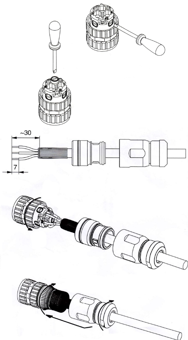
Rys. 8.15. Opis montażu przewodu ETH do konektora IP67
