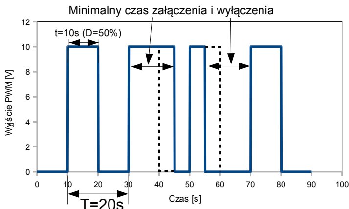
Rys. 7.101. Przykładowy przebieg wyjściowy przekaźnika typu OC w trybie PULSE
