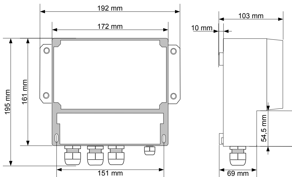
Rys. 4.3. Wymiary obudowy
