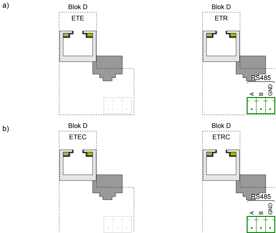
Rys. 4.13. Konfiguracje wejść dla Bloku D a) bez konektora IP67 na obudowie, b) z konektorem IP67 na obudowie
