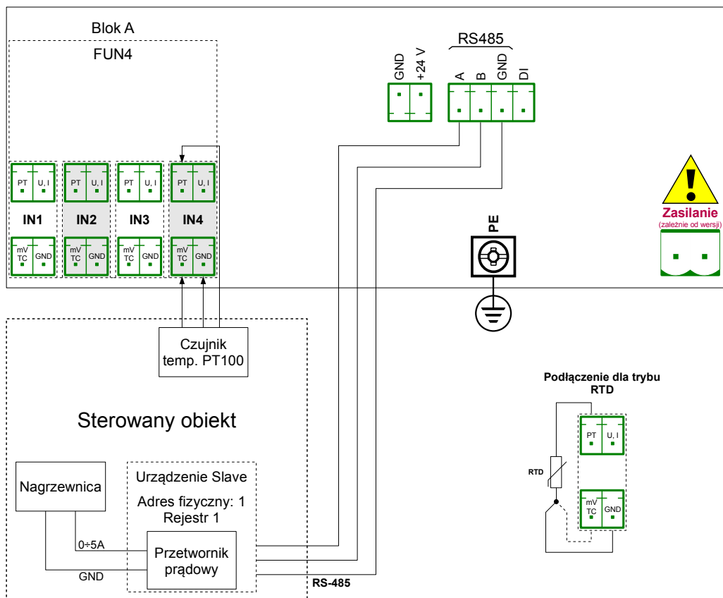
Rys. 7.85. Schemat połączeniowy dla konfiguracji sprzętowej FUN4 i portu Modbus MB1
