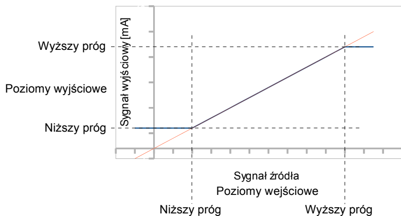
Rys. 7.103. Zależność sygnału wyjściowego (niebieski) od wejściowego (czerwony) dla Wyjścia prądowego
