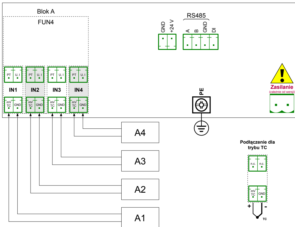
Rys. 7.79 Schemat połączeniowy dla sprzętowej konfiguracji wejściowej FUN4
