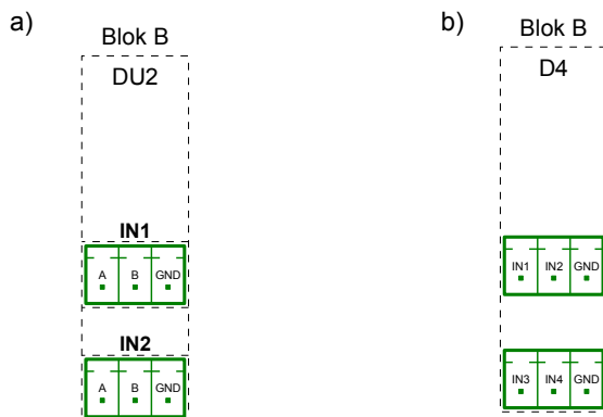
Rys. 8.7. Optoizolowane cyfrowe wejściowe konfiguracje sprzętowe dla Bloku B
