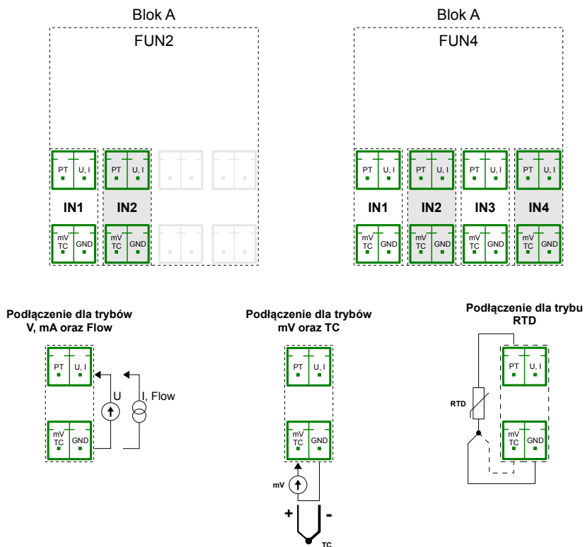
Rys. 8.2. Konfiguracje wejść dla Bloku A
