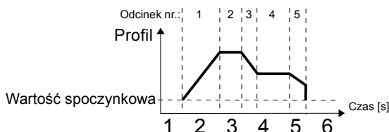
Rys.7.116. Przykładowy przebieg Profil/timera
