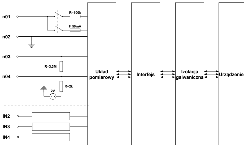
Rys. 8.3. Struktura wewnętrzna uniwersalnej wejściowej konfiguracji sprzętowej z funkcją przepływomierza
