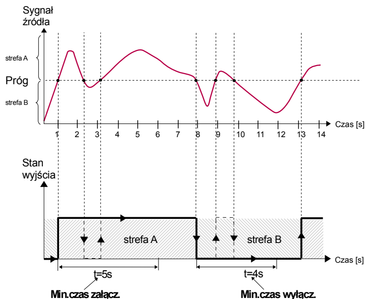
Rys. 7.98. Zasada pracy przekaźników wirtualnych dla przykładowych ustawień czasowych: Min.czas załącz. = 5 sec., Min.czas wyłączy. = 4 sec.
