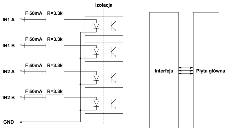
Rys. 8.8. Struktura wewnętrzna optoizolowanej konfiguracji sprzętowej DU2
