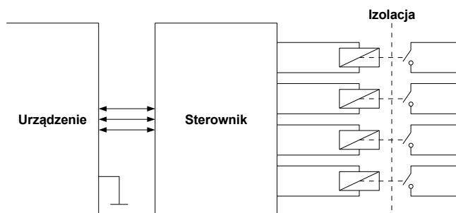
Rys. 8.13. Struktura wewnętrzna elektrycznych wyjść przekaźnikowych
