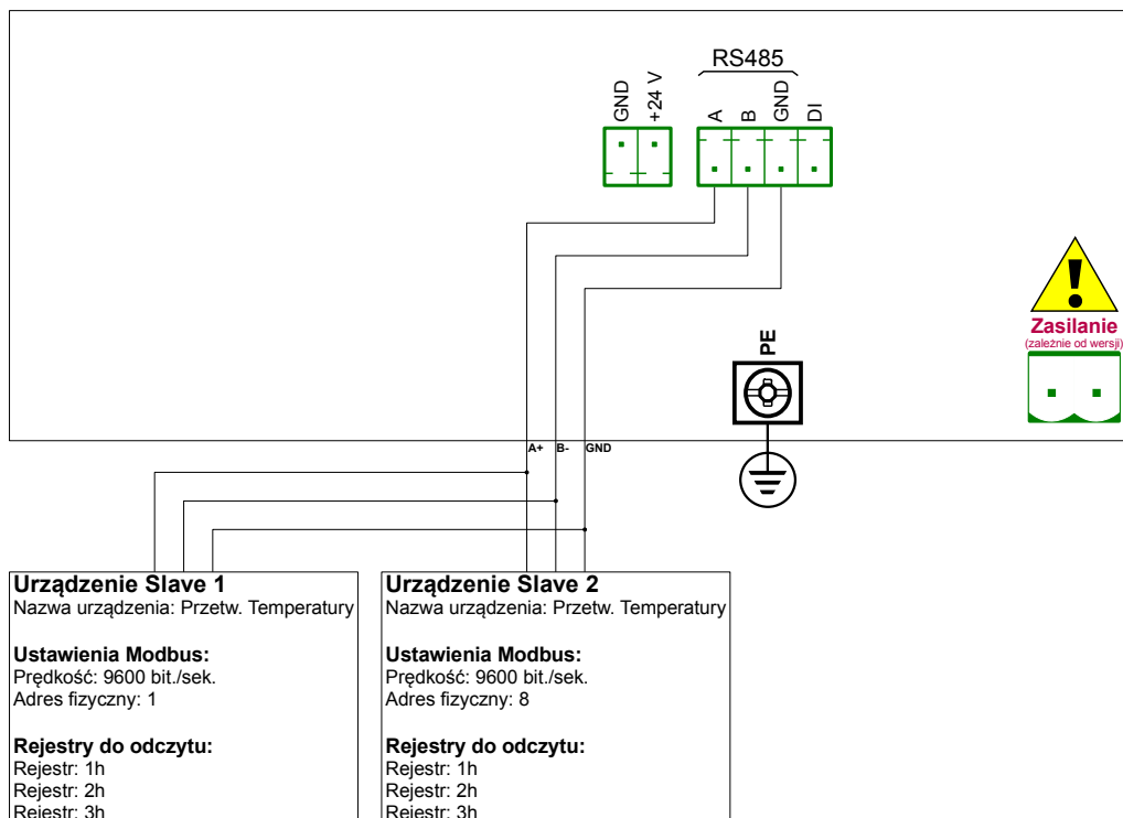
Rys. 7.83. Schemat połączeniowy dla portu modbusowego MB1
