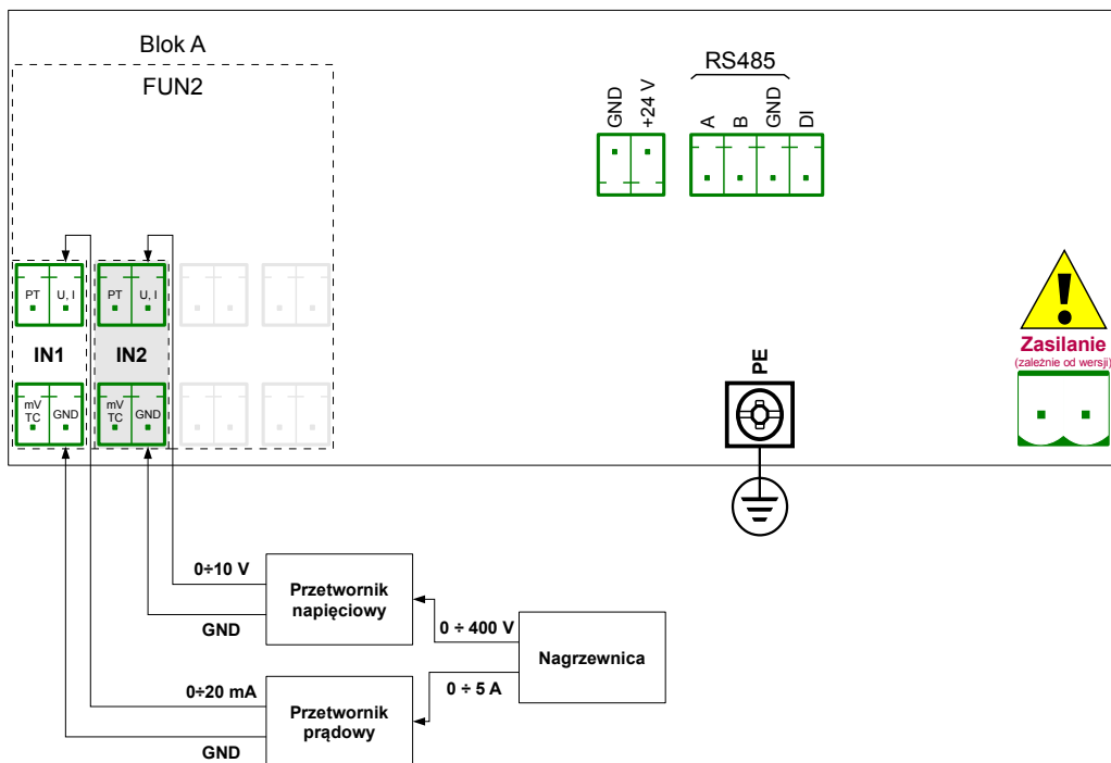
Rys. 7.73. Schemat podłączeniowy dla sprzętowej konfiguracji wejściowej FUN2
