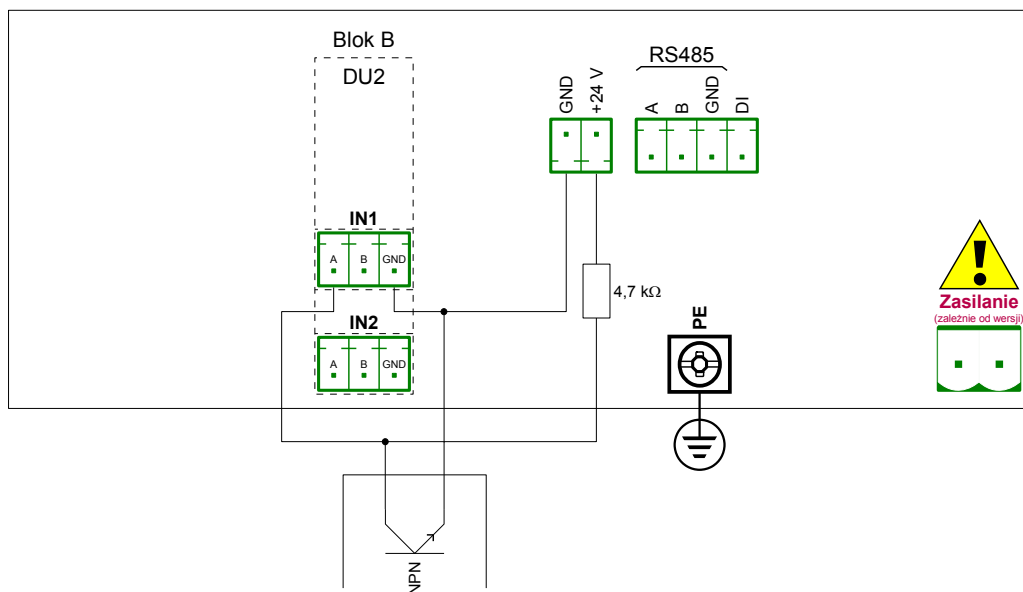
Rys. 8.11. Schemat podłączenia czujnika z wyjściem typu NPN do konfiguracji sprzętowej DU2
