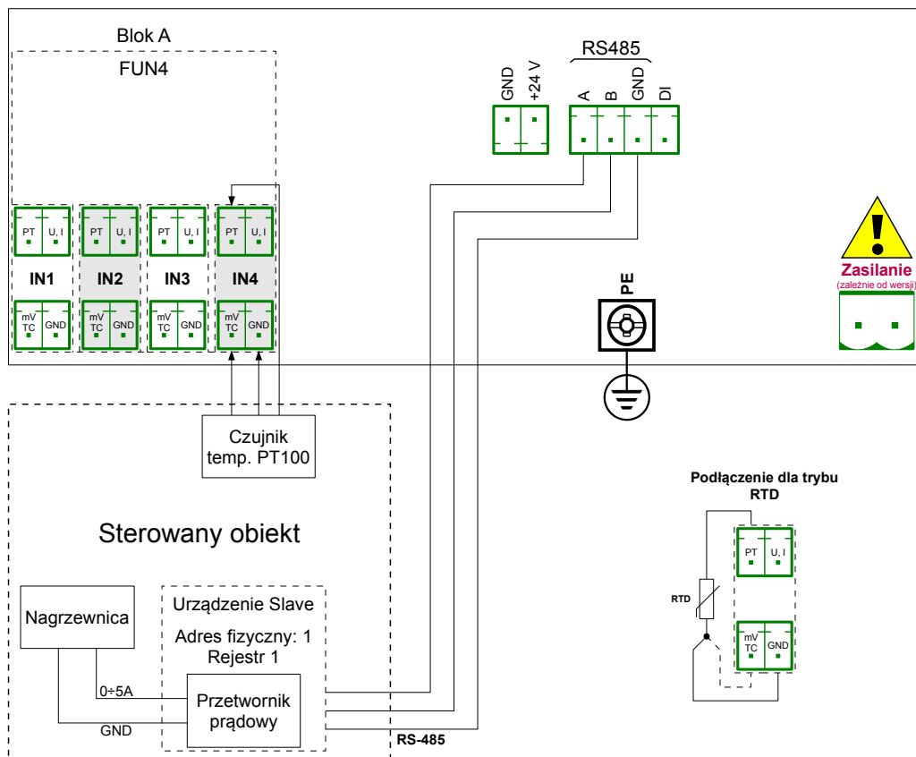
Rys. 7.137. Schemat połączeniowy dla konfiguracji sprzętowej FUN4 w trybie RTD i portu Modbus MB1
