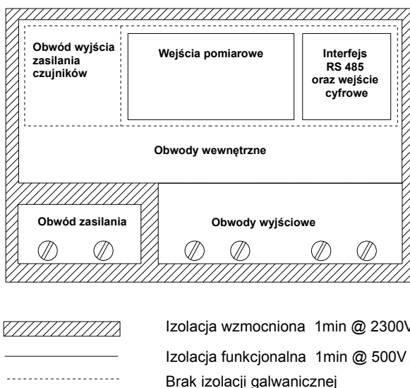
Rys. 4.1. Schemat izolacji pomiędzy poszczególnymi obwodami urządzenia
