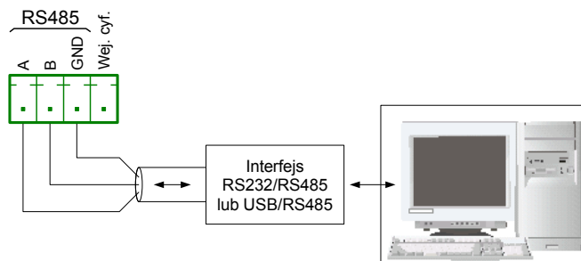
Rys. 4.14. Podłączenie sygnałów transmisji RS 485
