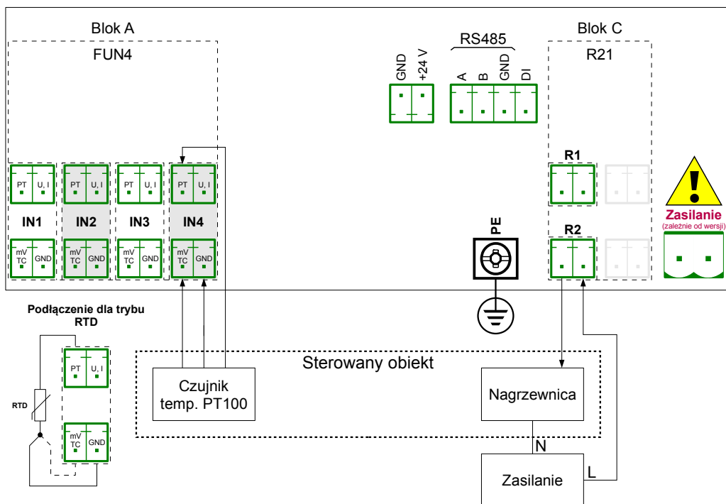
Rys. 7.105. Przykładowy sposób podłączenia do wejścia uniwersalnego w trybie RTD i wyjścia przełącznikowego
