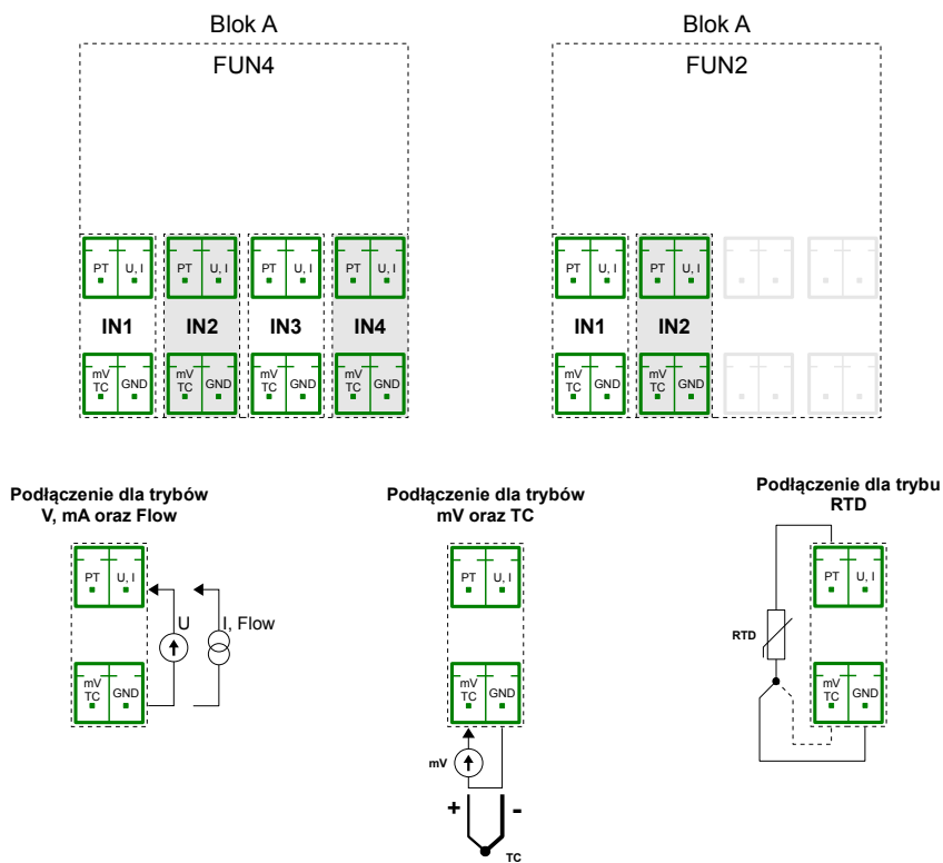
Rys. 4.10. Konfiguracje wejść dla Bloku A
