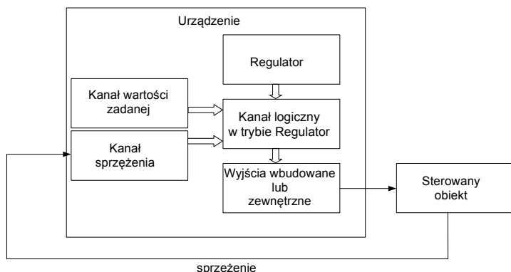
Rys. 7.127. Schemat blokowy procesu sterowania obiektem przy wykorzystaniu regulatorów
