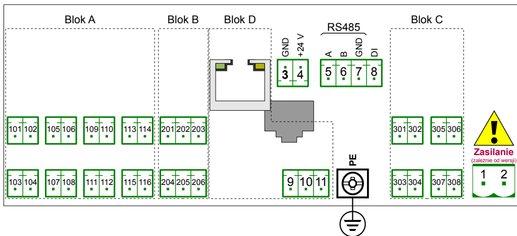
Rys. 4.8. Opis wyprowadzeń
