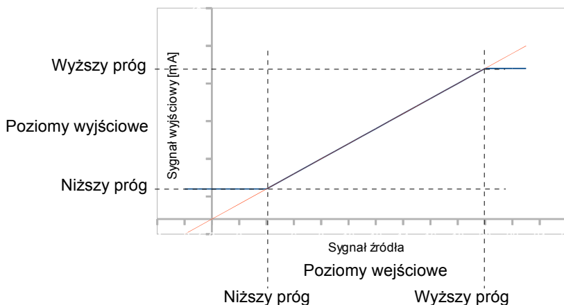
Rys. 7.110. Równanie transmisji (liniowe) sygnałów wejście - wyjście
