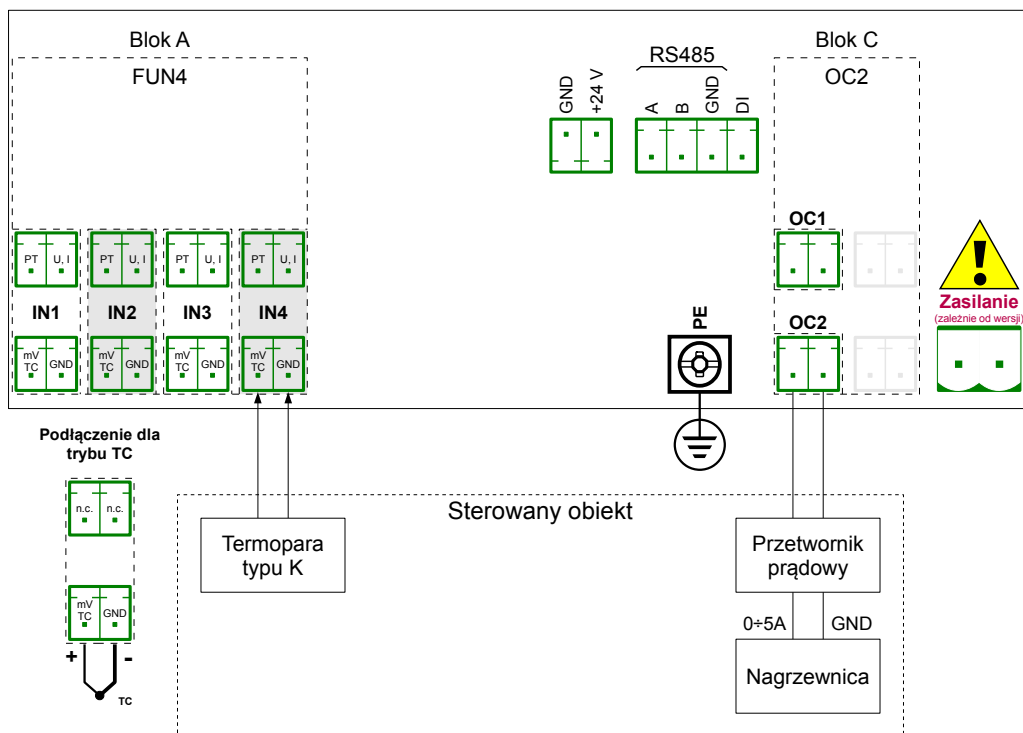
Rys. 7.138. Schemat połączeniowy dla konfiguracji sprzętowych FUN4 w trybie TC oraz konfiguracji sprzętowej OC2
