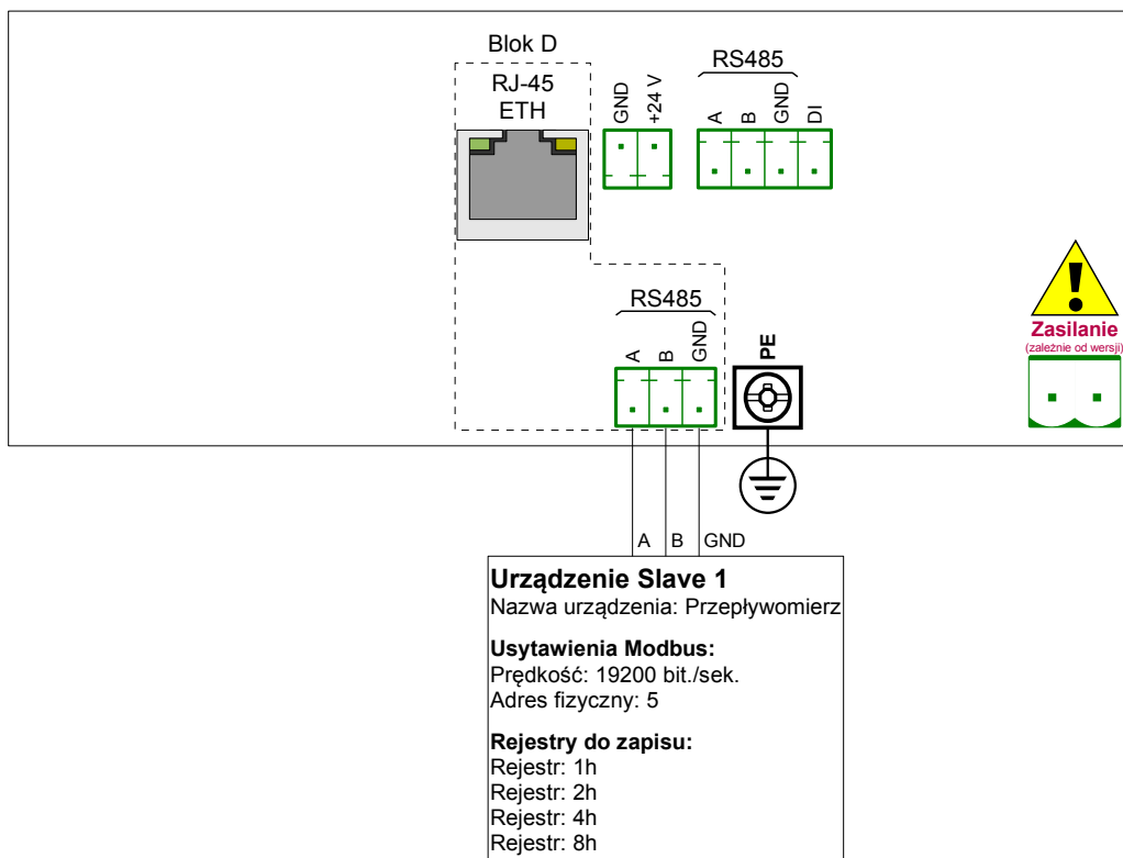
Rys. 7.168. Schemat połączeniowy dla portu modbusowego MB2
