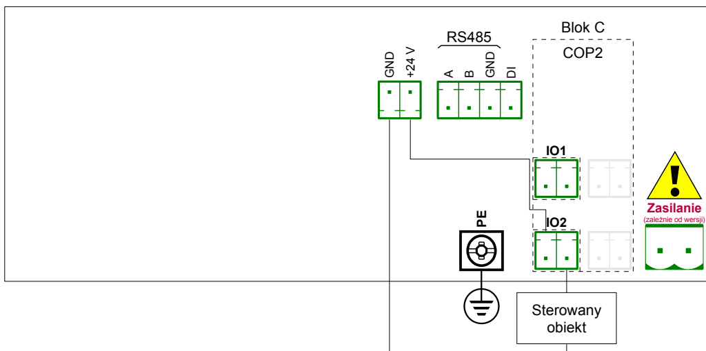
Rys. 7.106. Przykładowy sposób podłączenia pasywnego wyjścia prądowego
