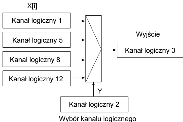
Rys. 7.84. Schemat blokowy działania funkcji matematycznej X[i] wybierane przez Y
