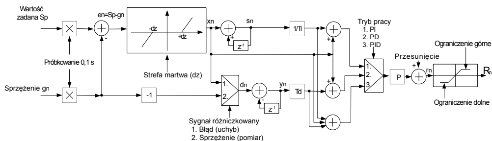
Rys. 7.128. Schemat blokowy Regulatora zaimplementowanego w urządzeniu
