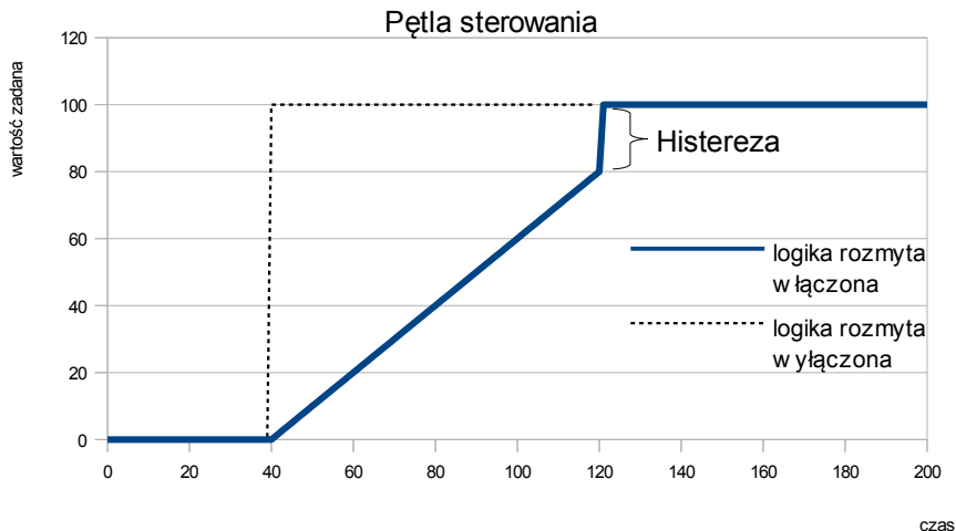
Rys. 7.126. Porównanie odpowiedzi regulatora na zmianę wartości zadanej przy wykorzystaniu i bez wykorzystania logiki rozmytej
