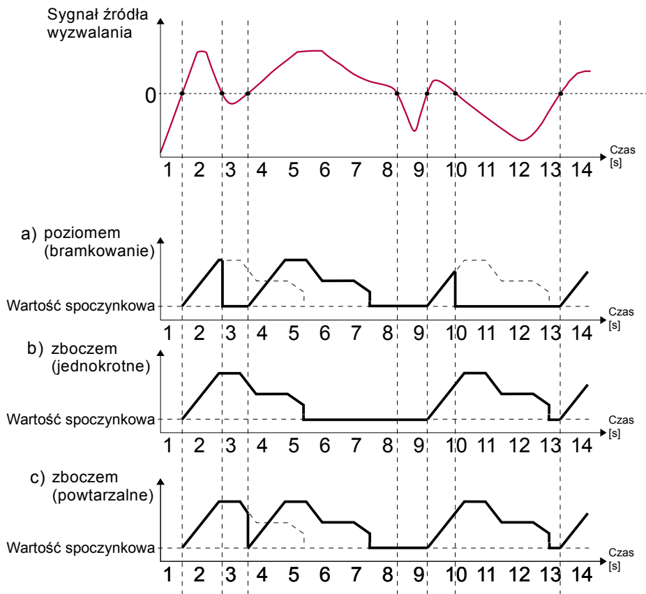
Rys.7.117. Przykładowe przebiegi wyjściowe Profilu zdefiniowanego na Rys.7.116 wyzwanego sygnałem źródła wyzwalania dla Trybu wyzwalania: poziomem (bramkowanie) , zboczem (jednokrotne) , zboczem (powtarzalne)
