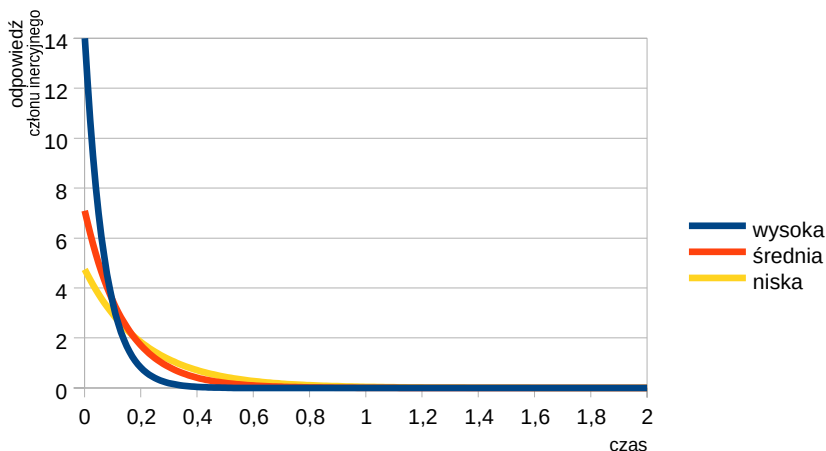
Rys. 7.124. Odpowiedzi układu inercyjnego w zależności od współczynnika T
