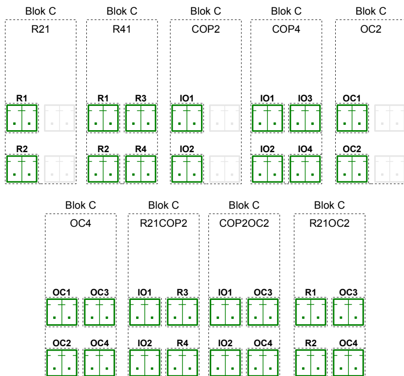
Rys. 4.12. Konfiguracje wejść dla Bloku C
