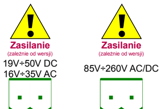
Rys. 8.1. Sprzętowe konfiguracje zasilające (od lewej): PS32, PS42
