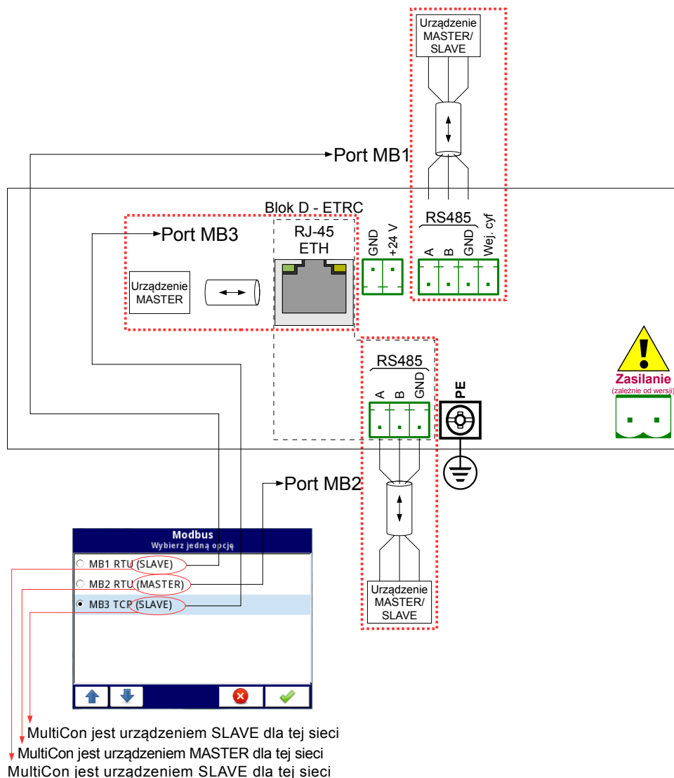
Rys. 7.63. Przykładowe podłączenie urządzenia MultiCon CMC-N16 w sieci z podglądem skonfigurowanych portów Modbus
