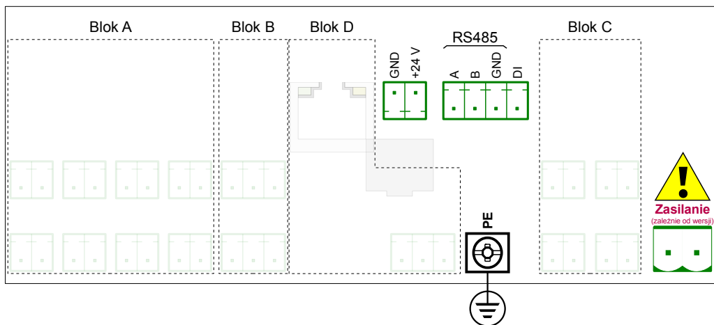
Rys. 4.9. Podstawowe wykonanie urządzenia
