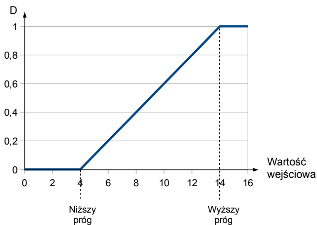
Rys. 7.100. Charakterystyka wejściowo - wyjściowa sygnału w trybie PULSE dla parametrów: Niższy próg=4 , Wyższy próg=14
