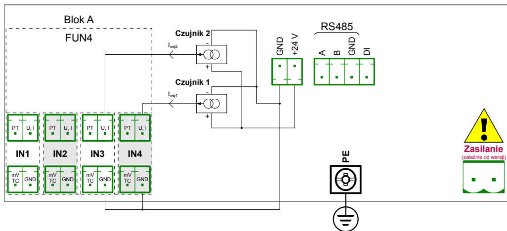
Rys. 8.5. Podłączenia przetworników prądowych 3-przewodowych
