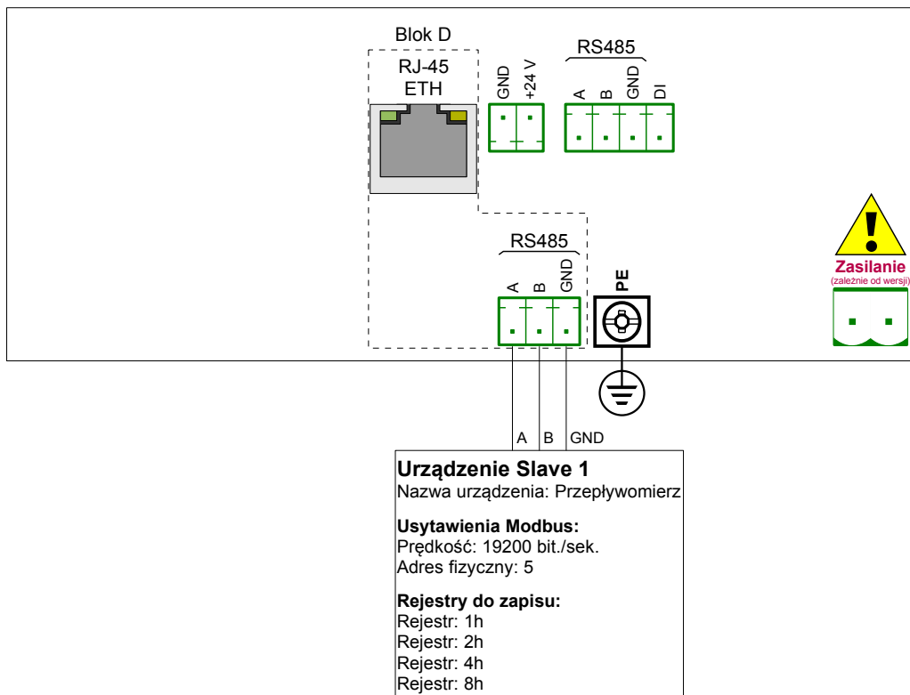
Rys. 7.111. Schemat połączeniowy dla portu Modbus MB2
