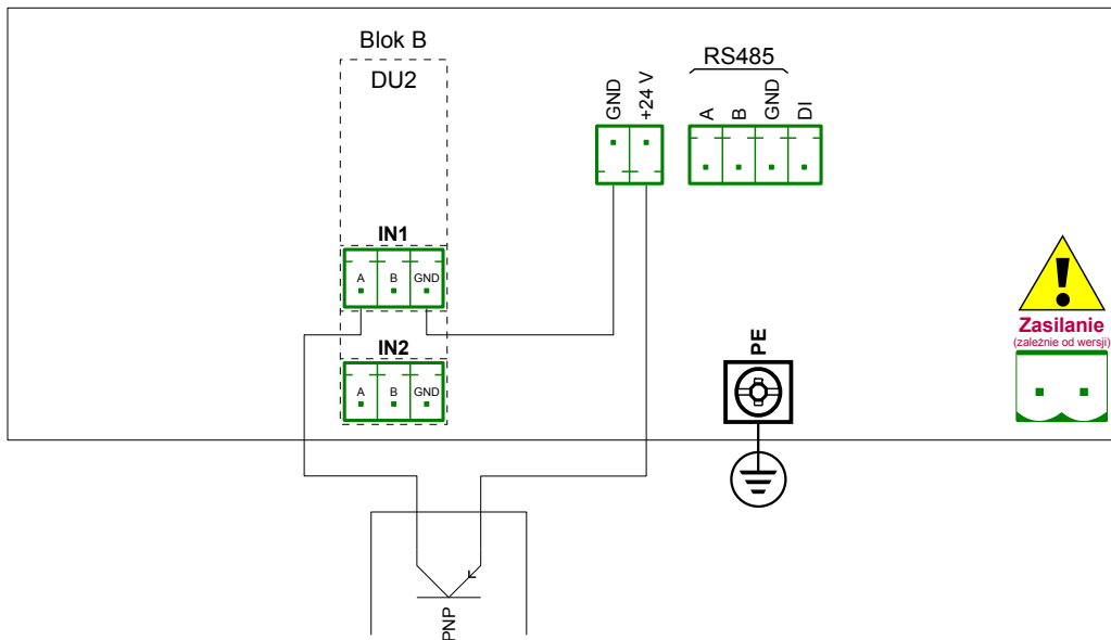
Rys. 7.87. Schemat podłączeniowy konfiguracji sprzętowej DU2 i czujnika typu PNP
