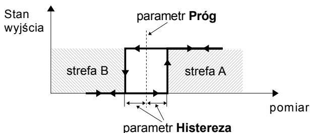
Rys. 7.94. Sterowanie jednoproęgowe przekaznika wirtualnego
