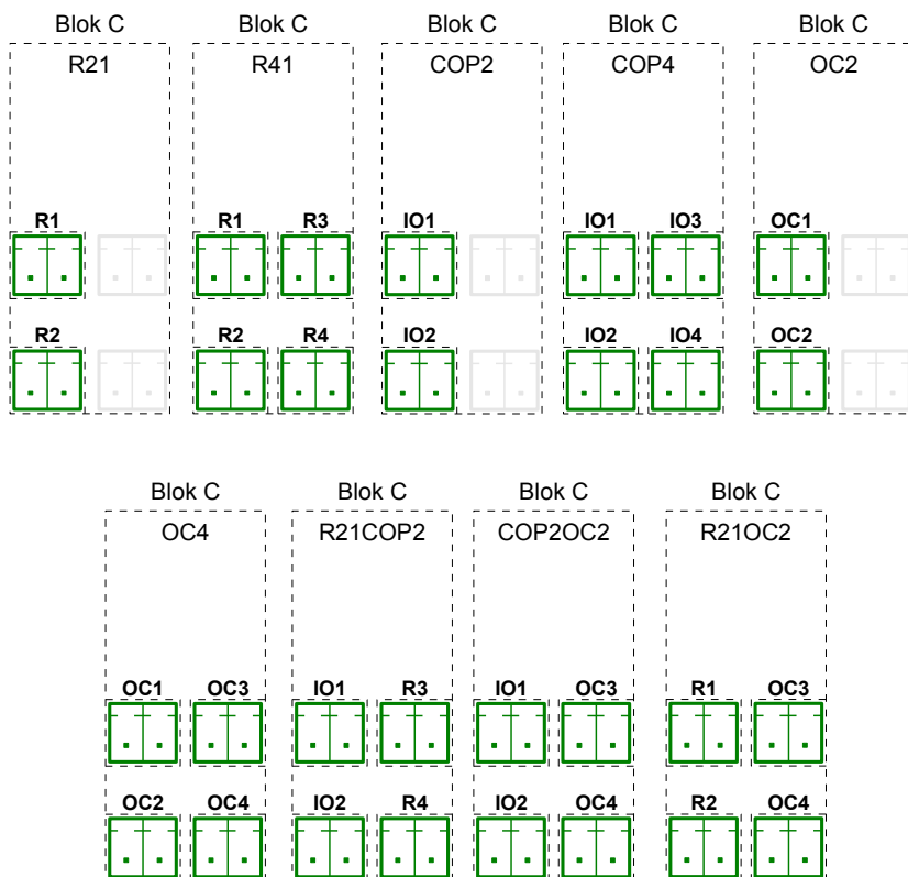
Rys. 8.12. Konfiguracje wyjść dla Bloku C
