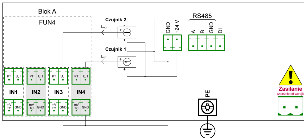
Rys. 8.6. Podłączenia przetworników napięciowych 3-przewodowych
