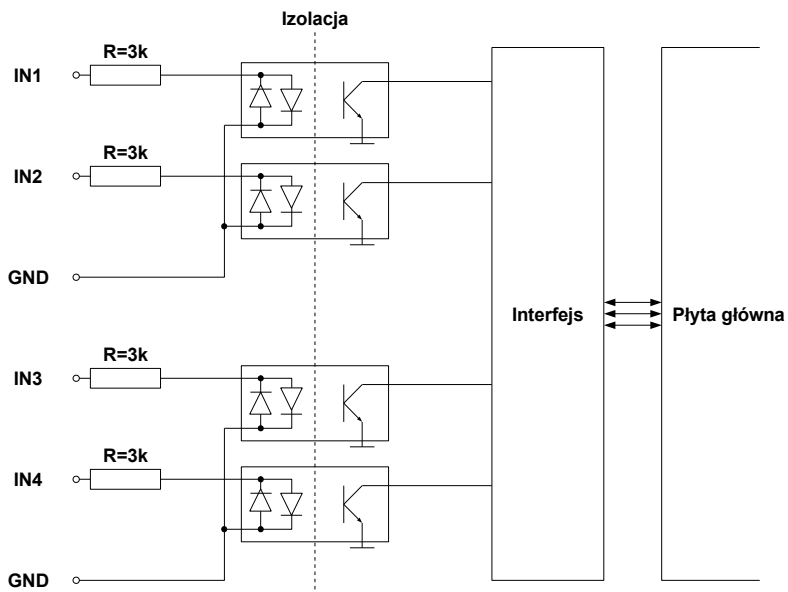
Rys. 8.9. Struktura wewnętrzna optoizolowanej konfiguracji sprzętowej D4
