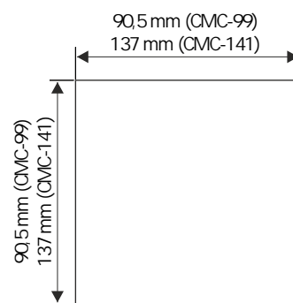
Wymiary otworu monta owego
