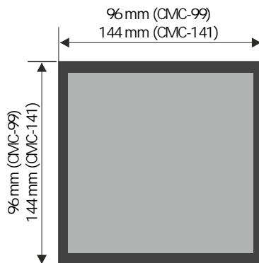
Wymiary zewn trzne
